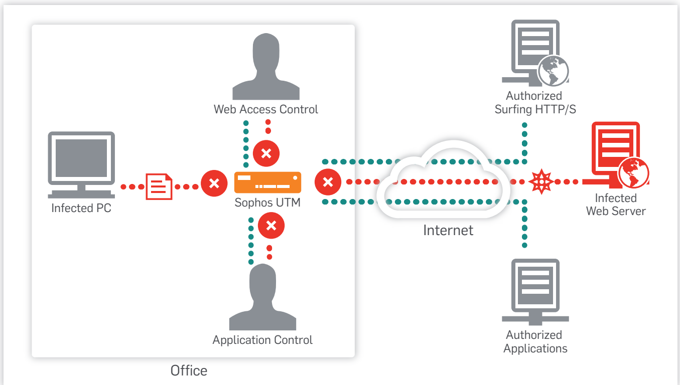
Einsatzszenario Sophos UTM Web Protection
