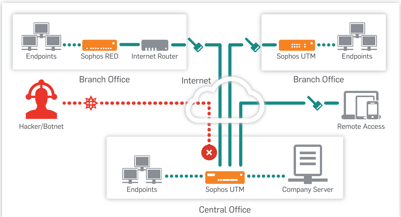
Einsatzszenario Sophos UTM Network Protection
